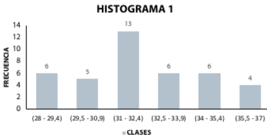
Figura 17. Ejemplo de histograma. Fuente: https://ikastaroak.birt.eus/edu/argitalpen/backupa/20200331/1920k/es/PPFM/GCPRLPA/GCPRLPA02/es_PPFM_GCPRLPA02_Contenidos/website_63_histograma.html
